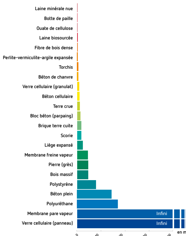
Sd moyen pour une épaisseur de 15 cm de matériau (hors membrane)
