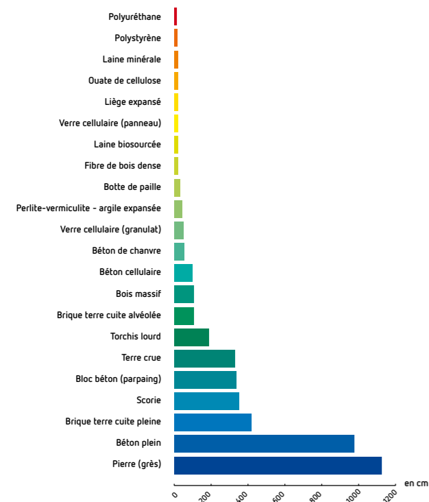
Épaisseur équivalente moyenne pour une résistance thermique R=5 m 2 .K/W
